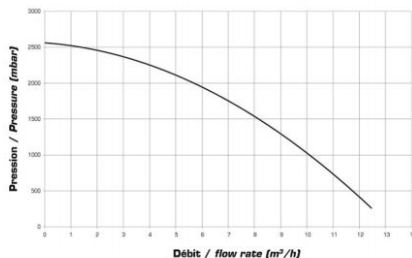
Course Supresseur - Performance Booster Pump
